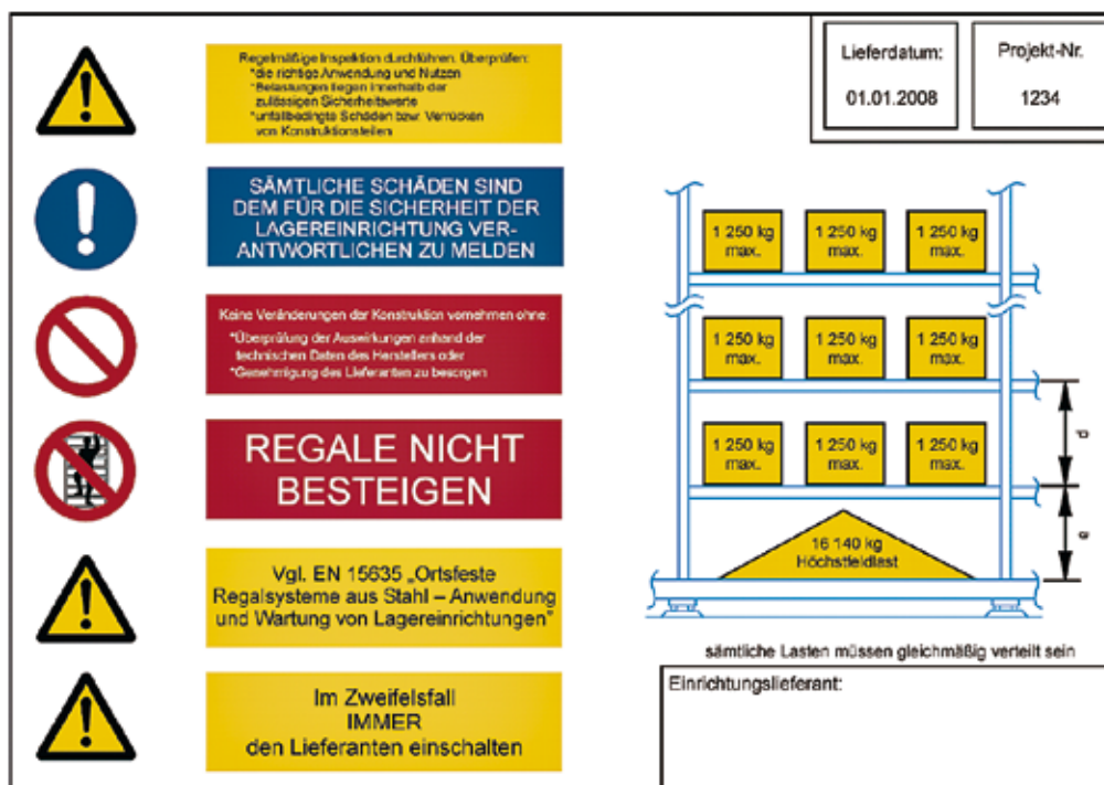
Abb. 16: Beispiel der Belastungsangaben für ein verstellbares Palettenregal, Abb. B.5 aus EN 1563
